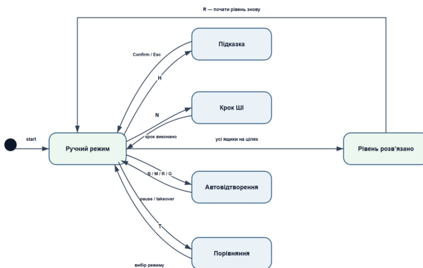
Рисунок Б.3 – Діаграма станів режимів взаємодії користувача та ШІ
