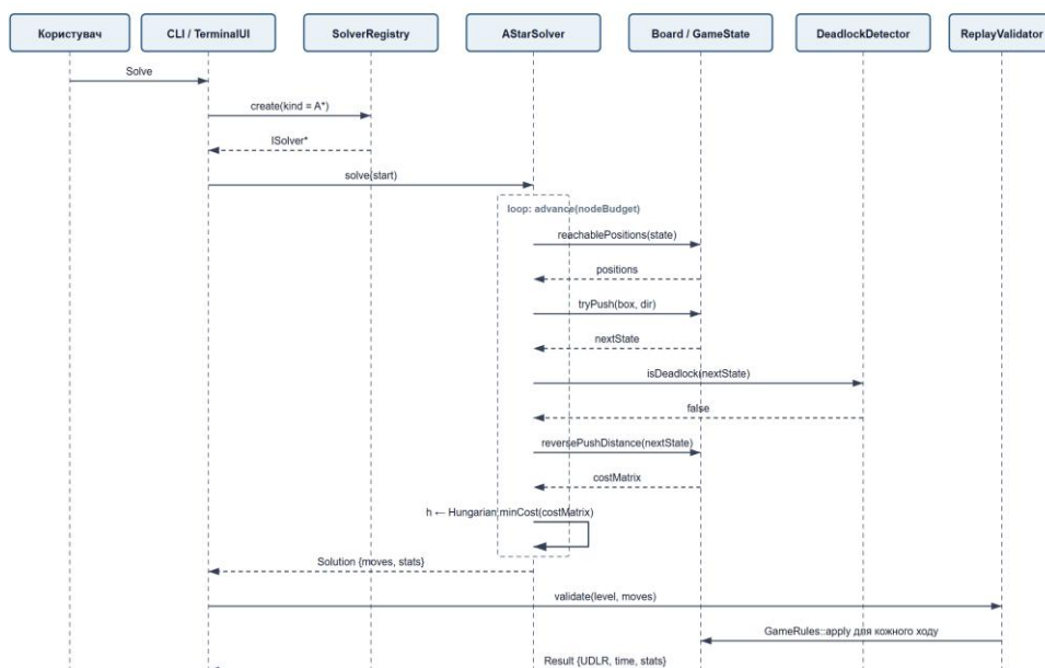
Рисунок Б.2 – Діаграма послідовності автоматичного розв’язання рівня
