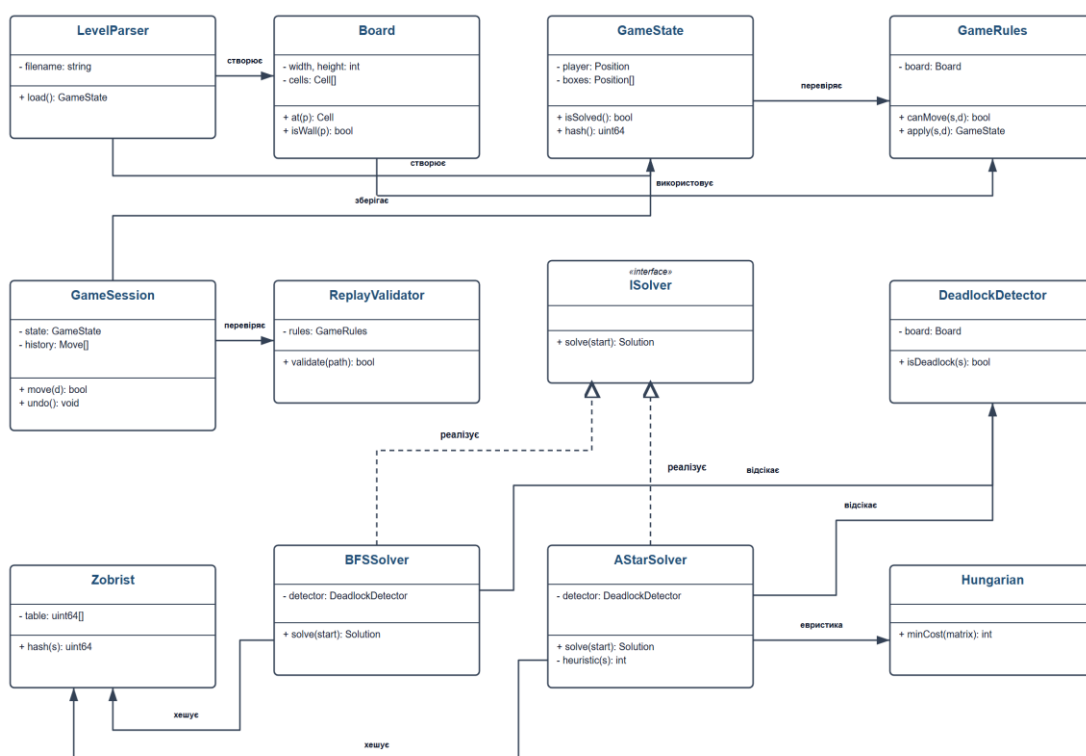
Рисунок Б.1 – Діаграма класів програмної системи «Сокобан»
