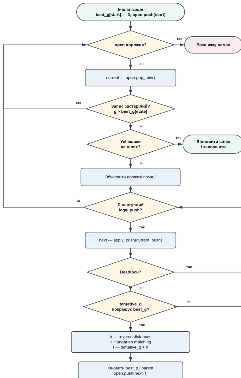
Рисунок 3.2 – Блок-схема алгоритму A*
