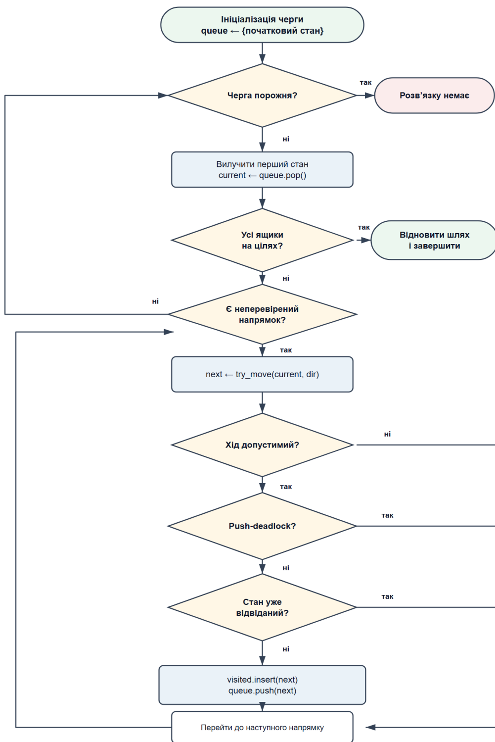
Рисунок 3.1 – Блок-схема алгоритму BFS
